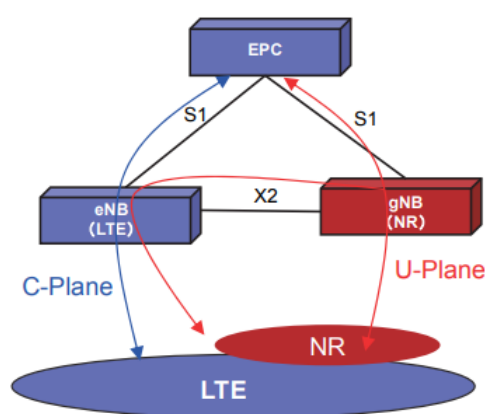
Fig. 4-8 LTE-NR Dual Connectivity接続イメージ
