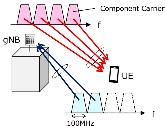
Fig. 4-7 ミリ波キャリアアグリゲーション (CA)
