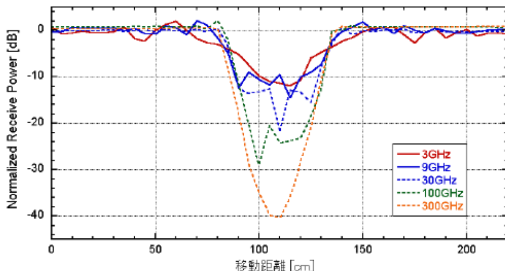
(Fig. 3-2 遮蔽ロスの測定結果例 [1])
