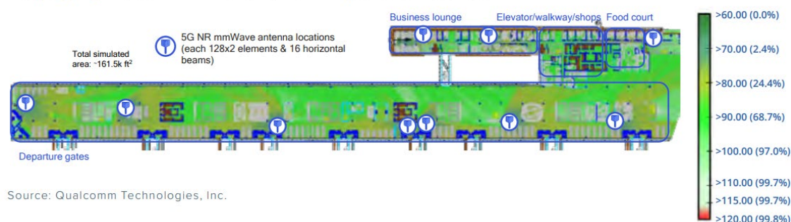
Fig. 5-5 空港における5Gミリ波基地局の設置例および伝搬損測定結果
