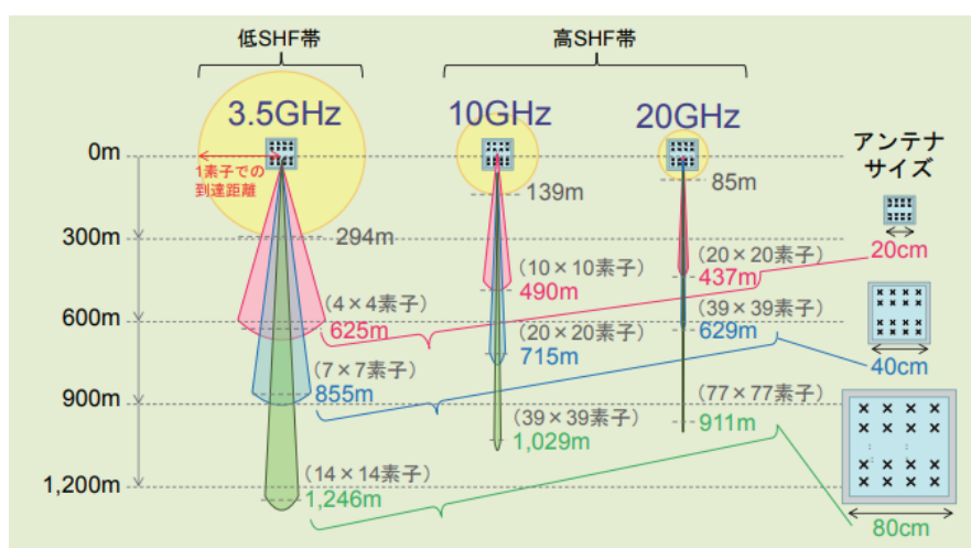
Fig. 4-2 ビームフォーミングの効果
