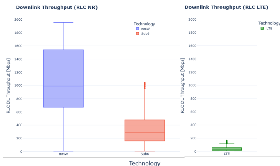
Fig. 5-8 屋外における5Gミリ波下りリンクスループット移動測定
