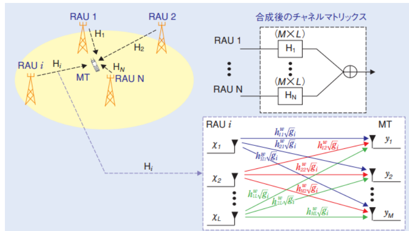
Fig. 4-3 送信機から受信機までのチャネルマトリックス
