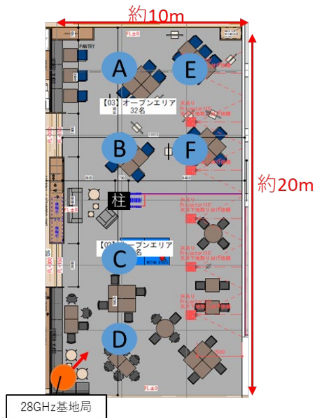
Fig. 5-4 5Gミリ波スループットの屋内測定
