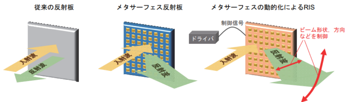
Fig. 4-4 メタサーフェス技術を用いたRISの概念図
