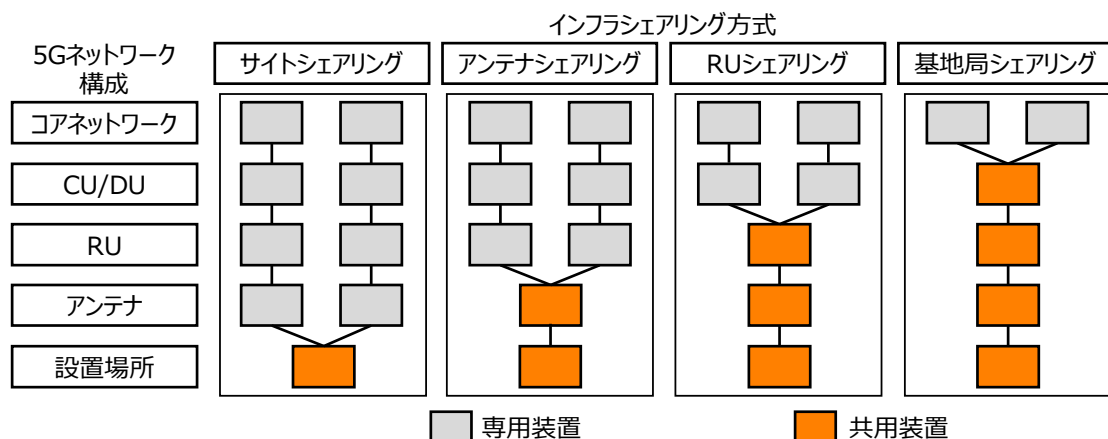
Fig. 4-6 インフラシェアリング方式の比較
