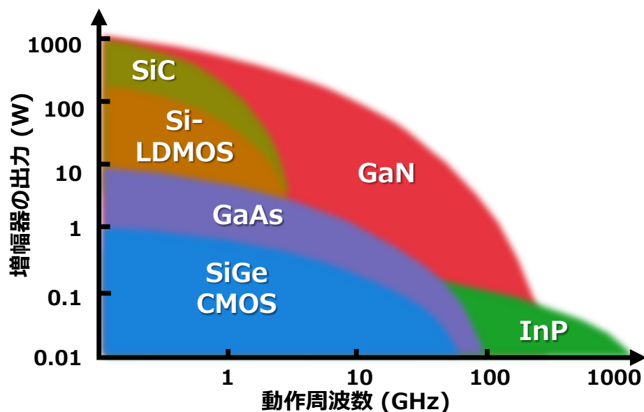
Fig. 4-5 周波数と増幅器出力の関係
