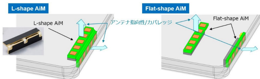
Fig. 9-5 Antenna Array Integrated Moduleの端末内配列 (村田製作所提供)
