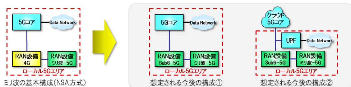
Fig. 7-6 ローカル5Gのミリ波におけるシステム構成例
