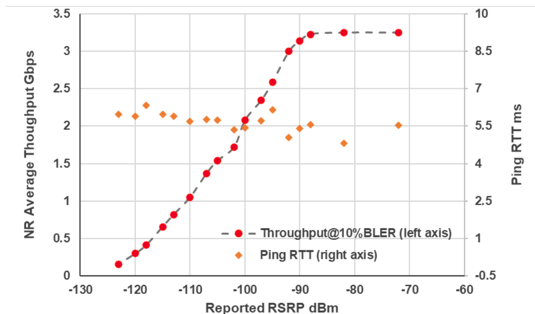
Fig. 5-3 5Gミリ波の端末受信スループットとラウンドトリップ遅延
