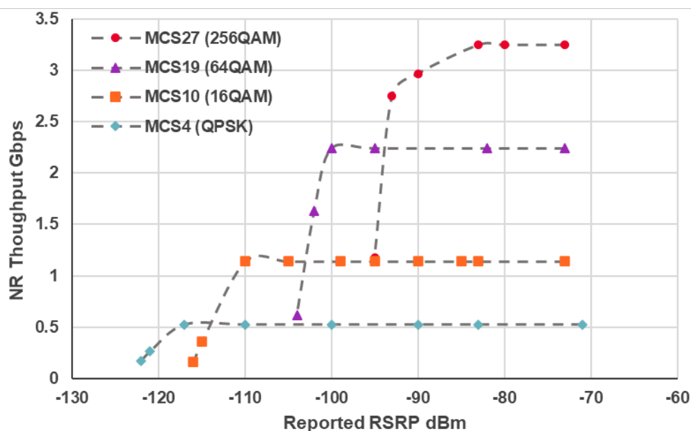
Fig. 5-2 5Gミリ波の端末受信スループット
