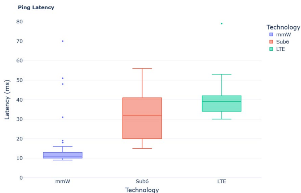
Fig. 5-9 屋外における5Gミリ波下りリンク遅延移動測定
