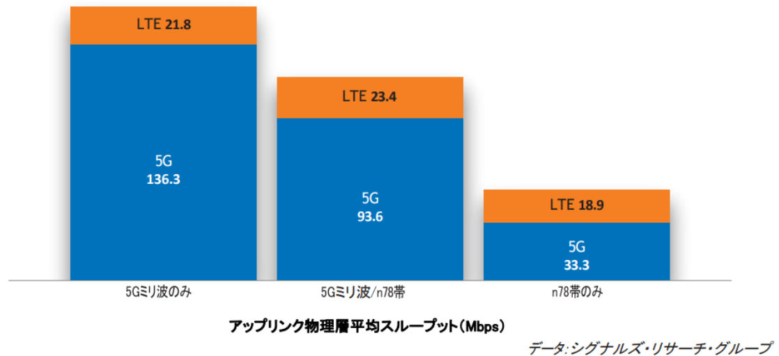
Fig. 5-7 屋外における5Gミリ波上りリンクスループット移動測定
